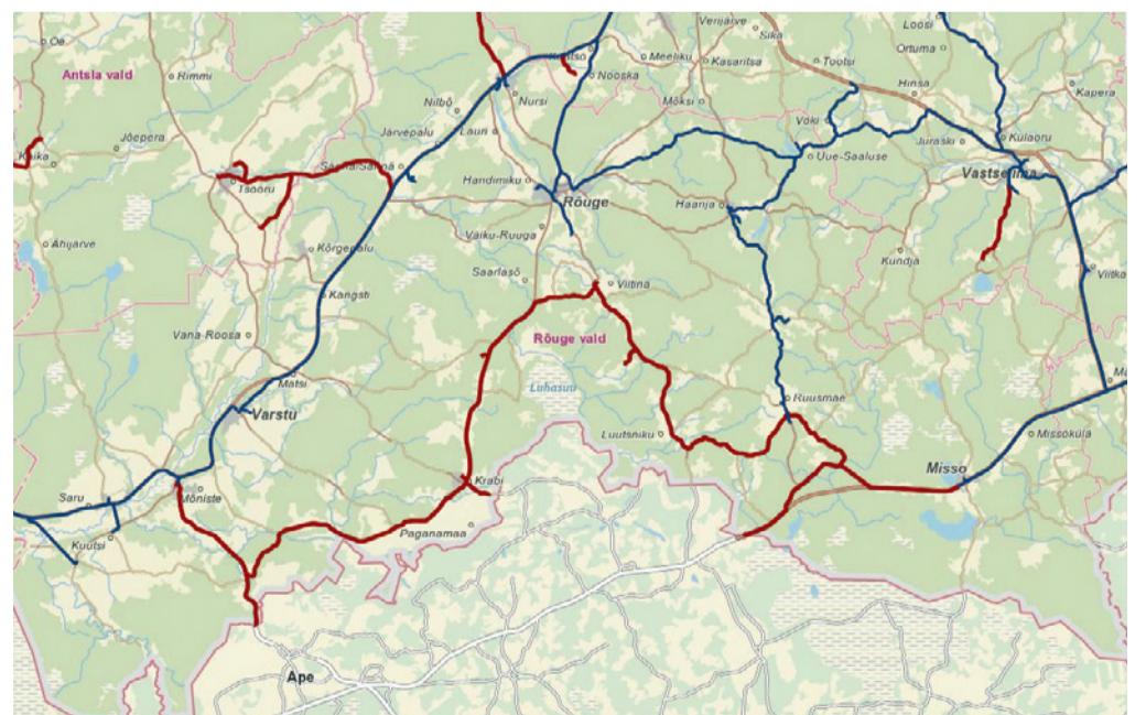
Rõuge valla piirkonnas ehitatud (sinisega) ja tänava ehitatav (punasega) EstWin baasvõrk (allikas: ELASA)
